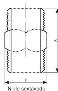
Figura 2931 - Niple para alta pressão - 3000 IBS - Neg 1 corpo Figura 2810 - Niple Sextavado em Aço Rosca BSP Figura 2820 - Niple Sextavado em Aço Rosca NPT Figura 2830 - Niple Sextavado em Aço Carbono BSP Figura 2840 - Niple Sextavado em Aço Carbono NPT
